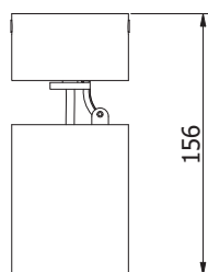
OS-FRG20W-10 OS-FRG20W-00
